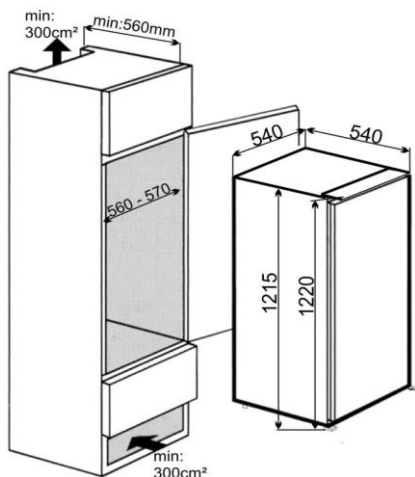
Einbauskizze
